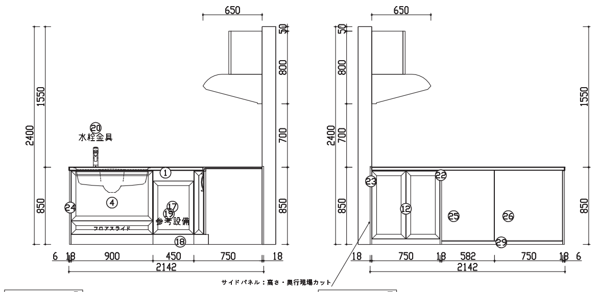
レイアウト展開図C
