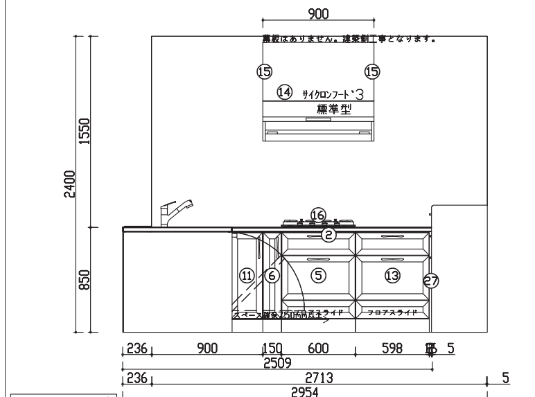
レイアウト展開図A
