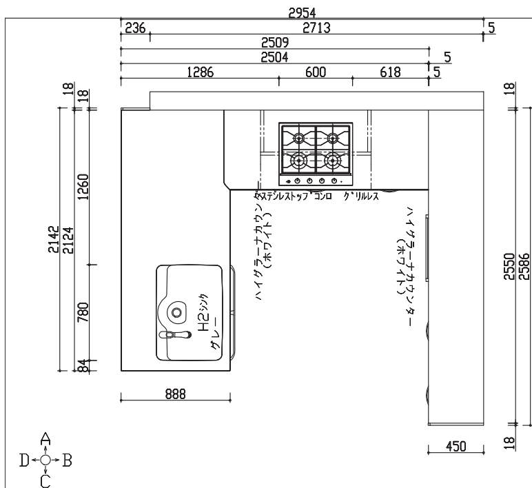
レイアウト平面図
